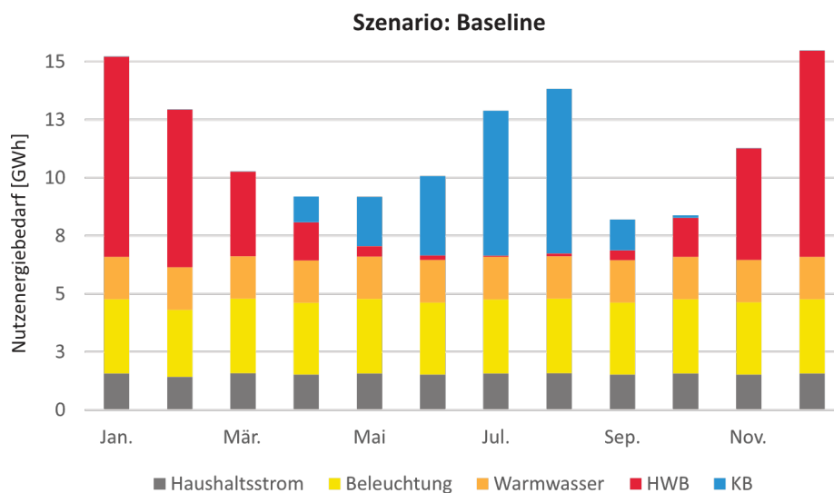
Abbildung 17: Darstellung des Nutzenergiebedarfs [GWh] des Baseline Szenarios ©IDUB
