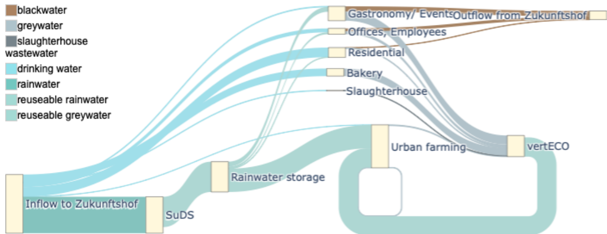
Abbildung 15: Darstellung der Ressourcenströme in Ausbaustufe 3: Wasser im August ©ANRI
