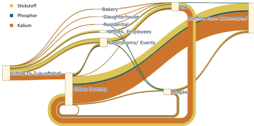
Abbildung 16: Darstellung der Ressourcenströme in Ausbaustufe 3: Nährstoffe im August ©ANRI
