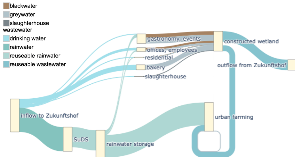
Abbildung 10: Wasserstrom am Zukunftshof (© KLIMUR)
