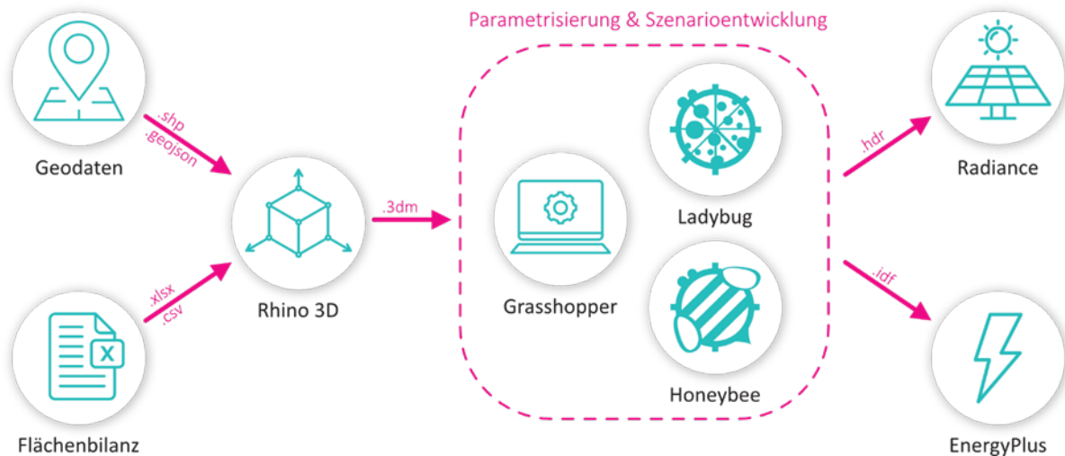
Abbildung 11: Schematische Darstellung des Workflows zur Erstellung und Bewertung der Szenarien für Rothneusiedl ©KLIMUR
