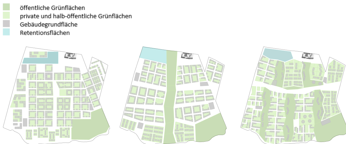
Abbildung 13: Konzeptübersicht der Szenarien (Baseline Variation – links, offene Mitte – Mitte, Durchwegung – rechts) © KLIMUR
