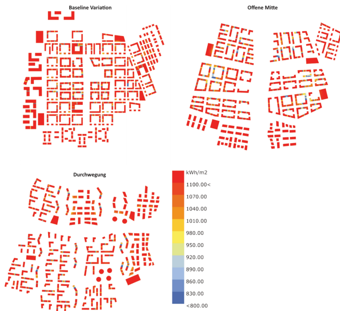
Abbildung 18: Grafische Darstellung des Solarpotentials der Entwicklungsvarianten.
