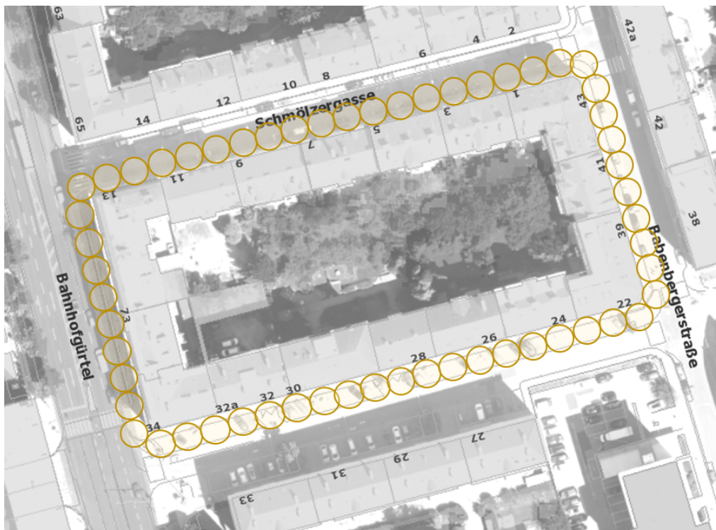
Abbildung 15: Visualisierung der maximal zur Verfügung stehenden öffentlichen Flächen für die Abschätzung des Geothermiepotezials inkl. Darstellung der maximal möglichen Sondenanzahl bei einem Sondenabstand von 7 m
