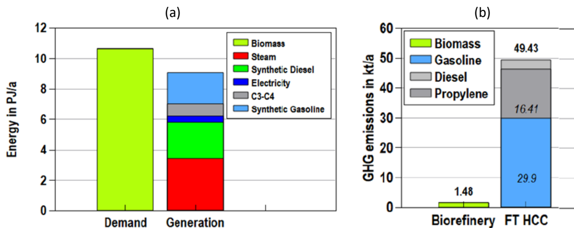
Abbildung 4: Ergebnisse der TEE- Bewertung hinsichtlich (a) Energieeffizienz und (b) Treibhausgasemissionen betreffend der Bioraffinerie mit Vergasungs- und FT-Prozessen (mit FCC-Verarbeitung), (Quelle: Lindorfer et al., 2022)
