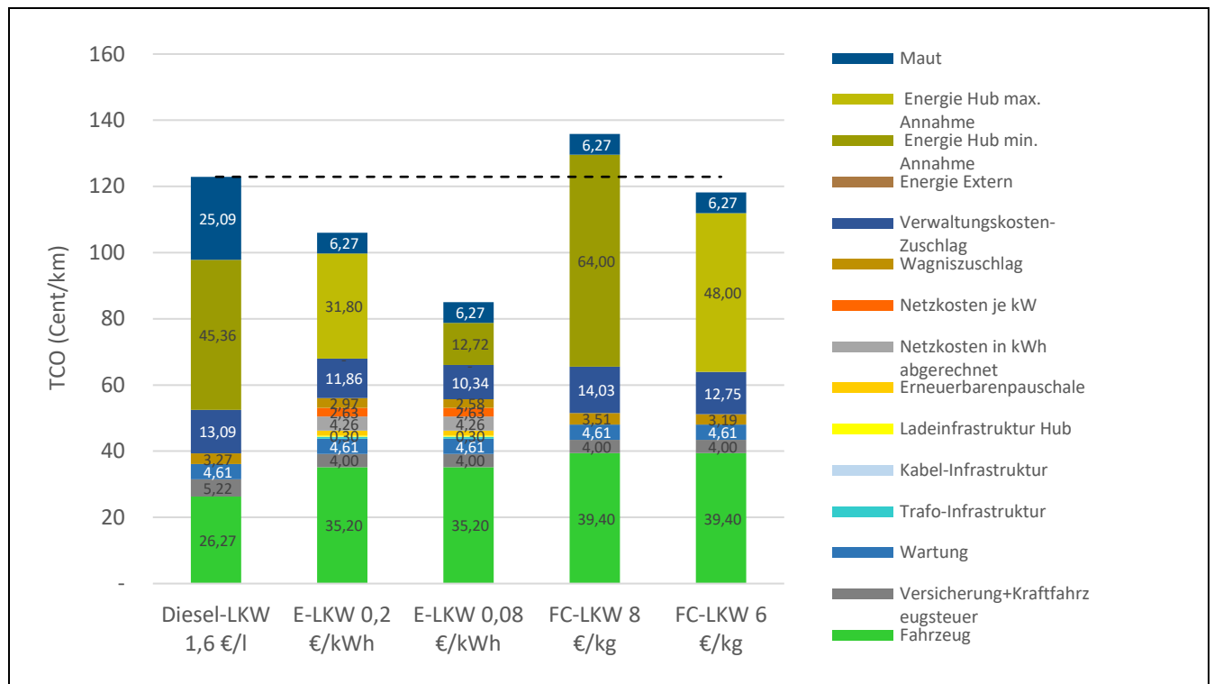
Abbildung 7: TCO von Diesel-/E-/FC-LKW unter verschiedenen Preisannahmen (Use Case: Logistik)
