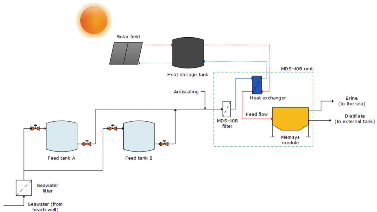
Abbildung 14: Pilotanlage für die Meerwasserentsalzung basierend auf einer Vakuum-MEMD versorgt über Solarthermie (21)
