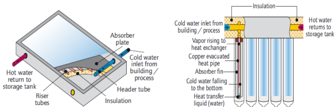
Abbildung 10: Flachkollektor (links) und Vakuumröhrenkollektor (rechts) (20)
