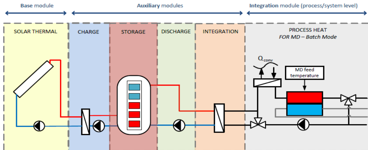
Abbildung 12: Übersicht über ein Integrationskonzept – Solarthermie zur Versorgung der Membrandestillation
