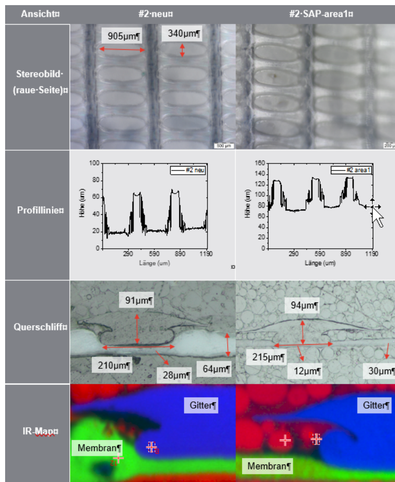
Abbildung 1: Illustration der PP-Gitter- und PTFE-Membranstruktur eines beispielhaft untersuchten MD-Funktionselementes im Referenzzustand (links) und nach Einsatz (rechts).
