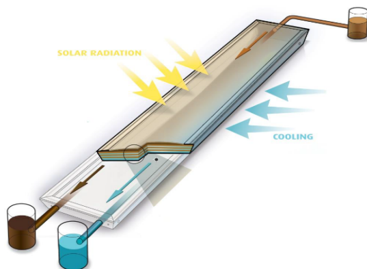
Abbildung 5: Aufbau des Kollektors von SOLARDEW (siehe Fußnote 4)
