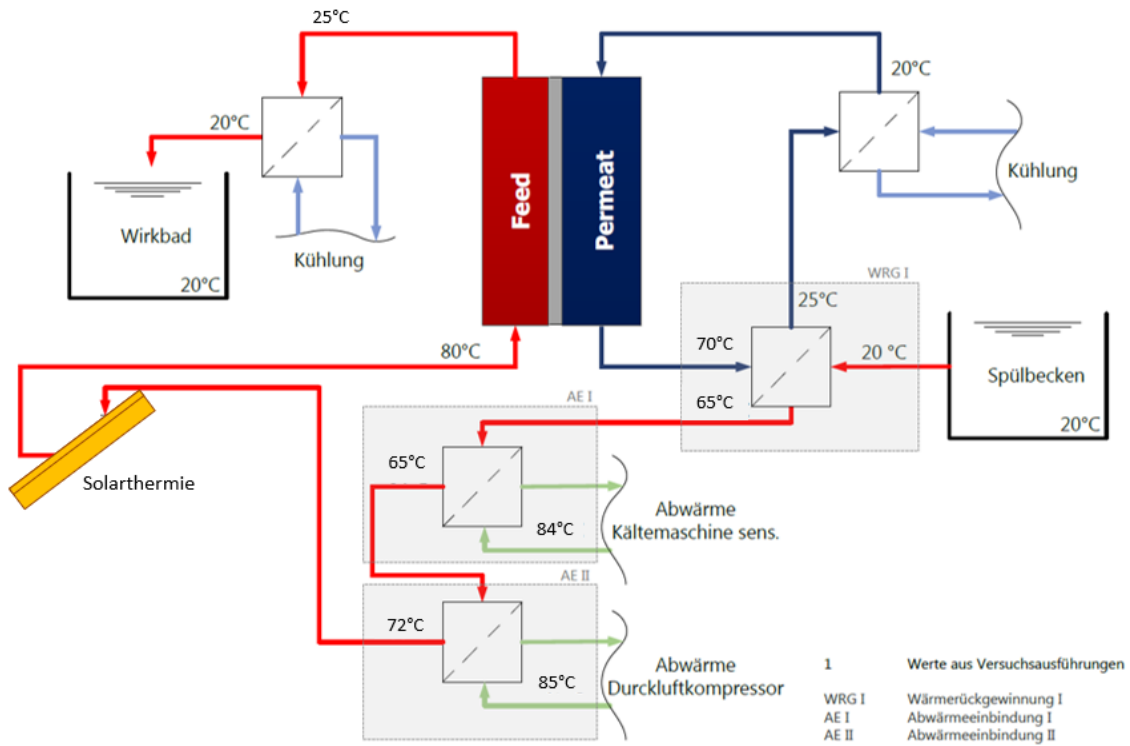
Abbildung 13: Integrationskonzept für die Versorgung der Membrandestillation mit Abwärme und Solarthermie (parallel)
