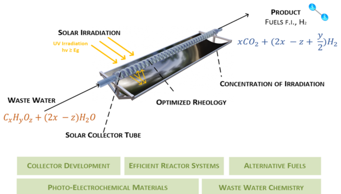
Abbildung 9: Aufbau des Solarreaktors(AEE INTEC)
