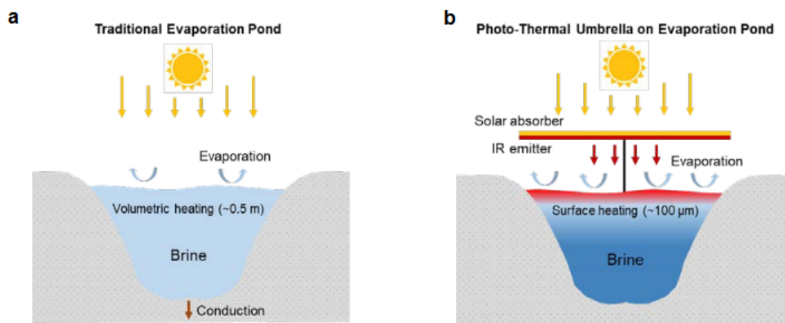
Abbildung 3: Darstellung des solaren Teiches mit dem photo-thermischen Schirm (14)
