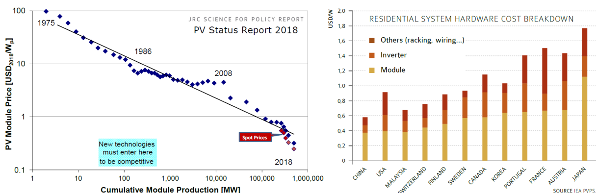
Abb. 5: Links: Preisentwicklung (Lernkurve) für den Weltmarktpreis von PV-Modulen [37]. Rechts: Kosten für Haus-PV-anlagen einiger Länder [29].
