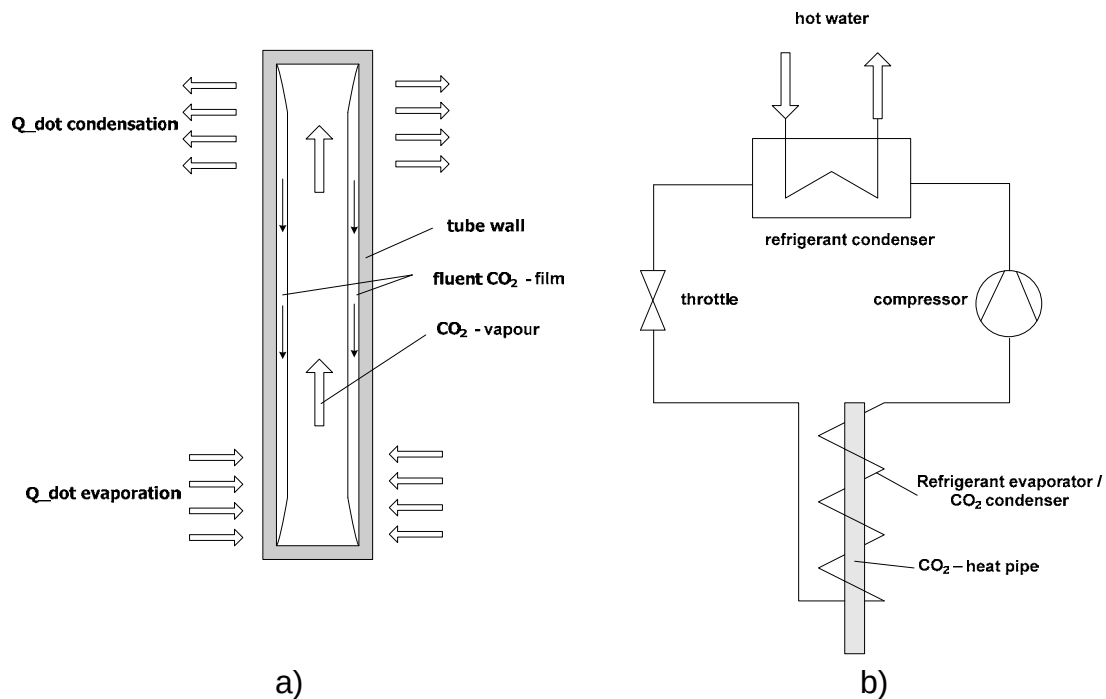
Abbildung 11: CO 2 -Wärmerohr
