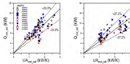
Q vs. UA für R407C BW mit \Delta T_{\text{sink}}=5\text{K} für den Nassdampfgebiet in Kondensator und Verdampfer
